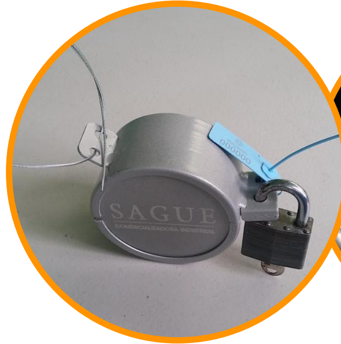
Cuenta con orificios para sello de seguridad, candado y para sujetar al tanque.
