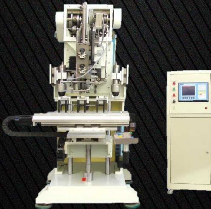
MÁQUINA DE BARRENADO E INSERTADO DE CEPILLO 2 EJES MOD. GS403Z
