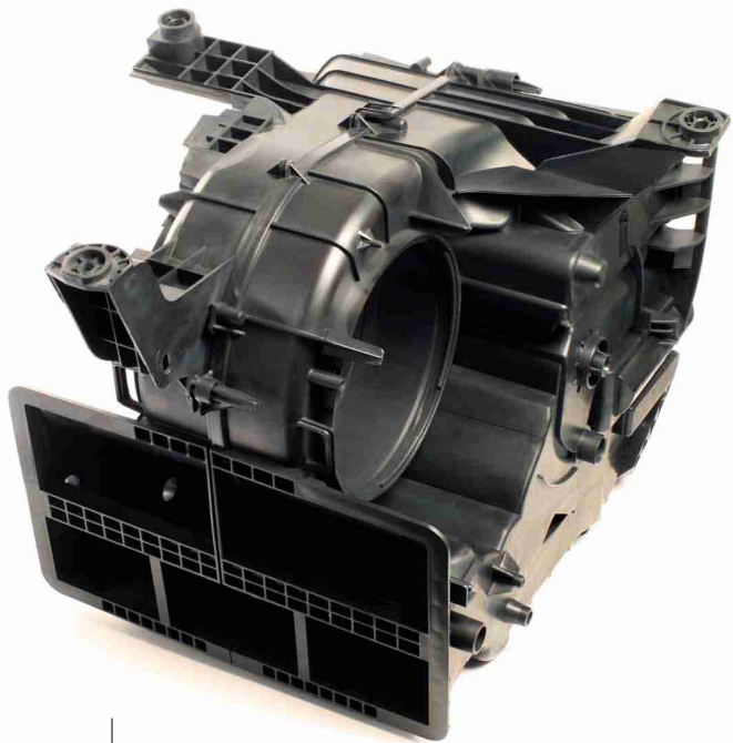
Distribuidor de aire acondicionado (molde 12T). Industria automóvil.
