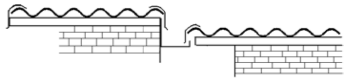
Fijación del flashing al muro
