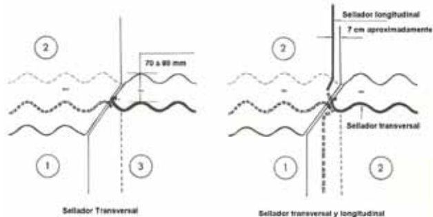
Sobre traslape transversal
