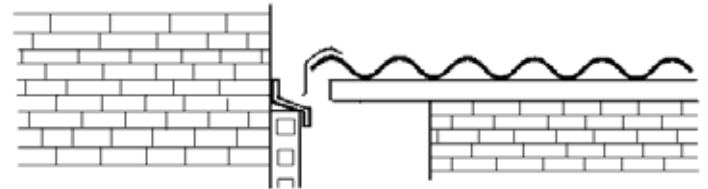
Fijación del flashing al muro
