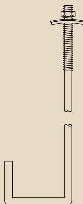
Bilro para hacer el dobles, con tuerca hexagonal y arandela con EPDM
