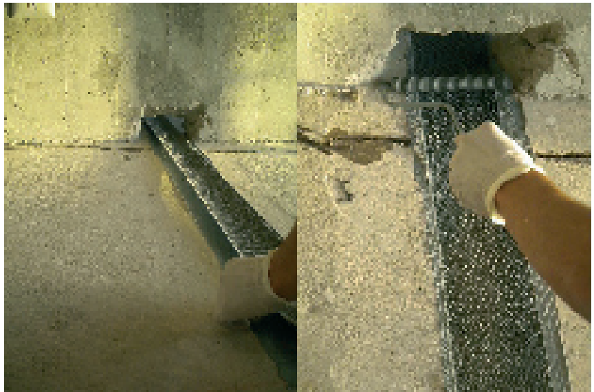
Reforzamiento de losa de entpiso en lecho superior con SikaWrap 300 C Z..
