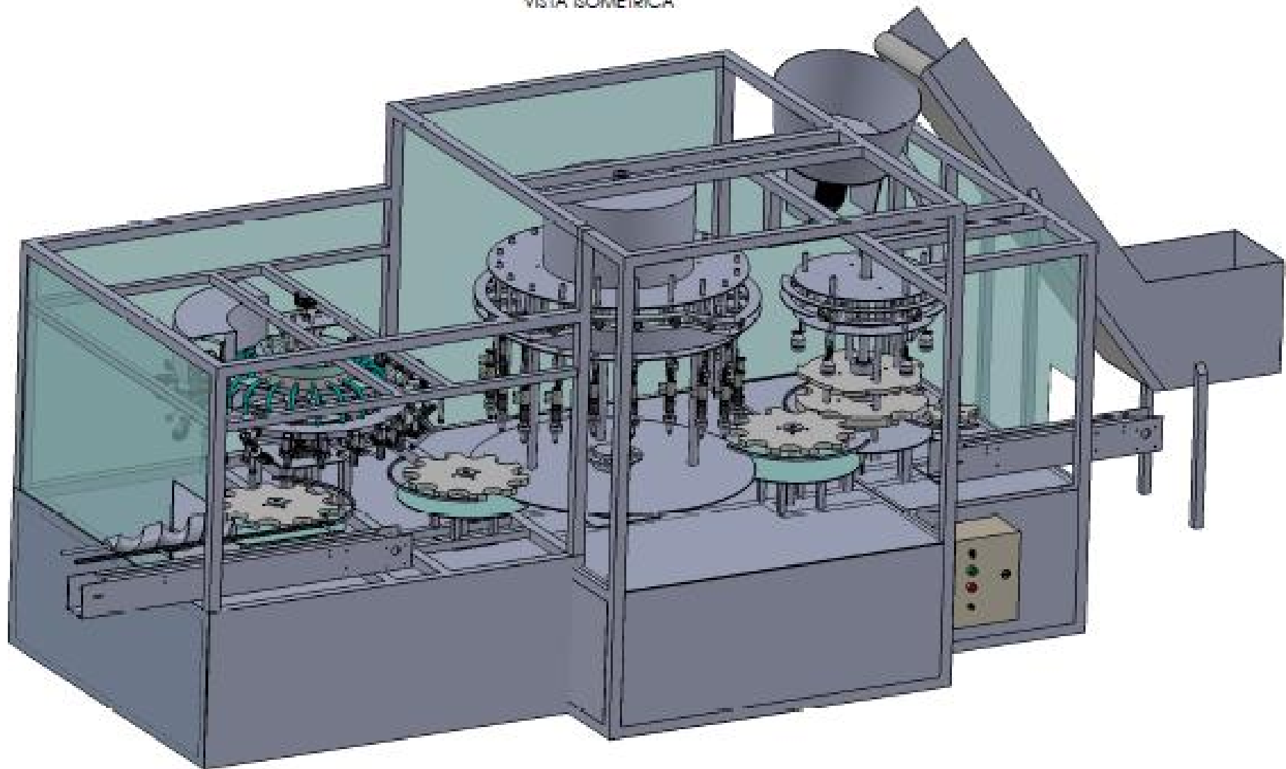
TRIBLOCK (ENJUAGADO LLENADO Y TAPADO)
